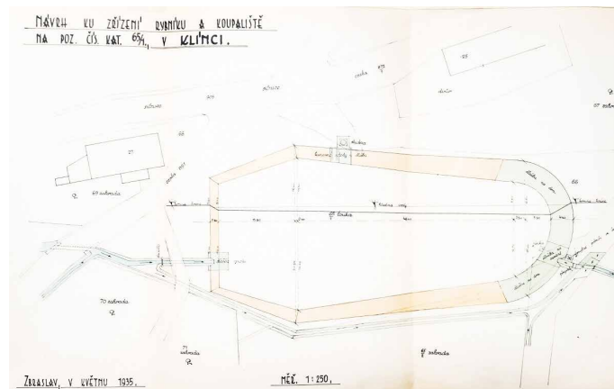
Plánek z roku 1935. Podnikatelství staveb František Vodička, Zbraslav.
